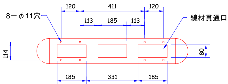
平面図(下)
