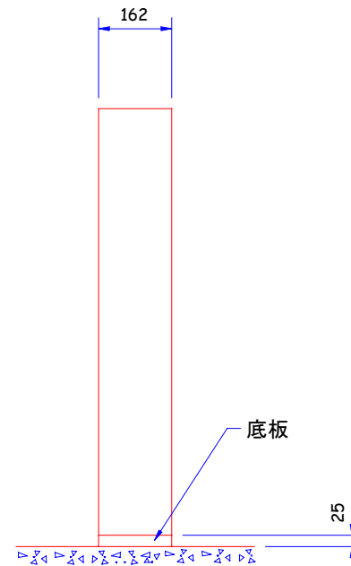
端面図
