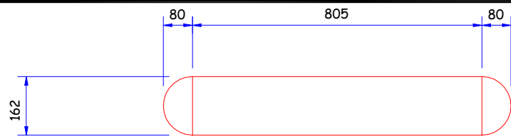
平面図(上)
