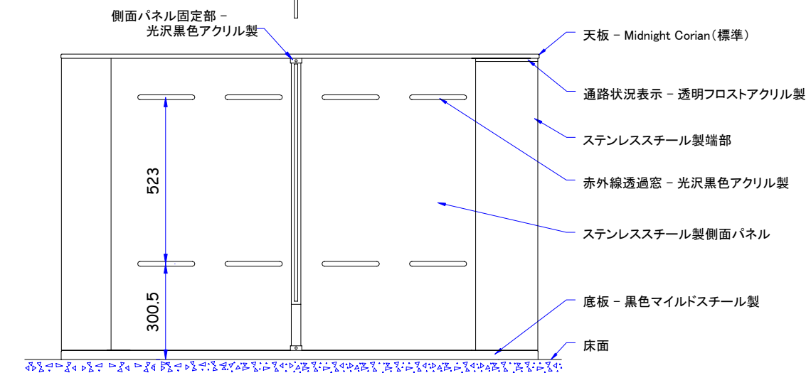
側面図
