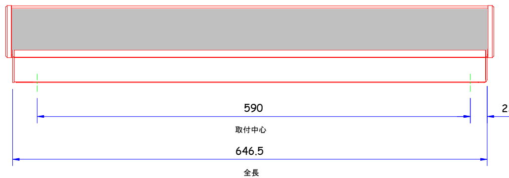
側面図
