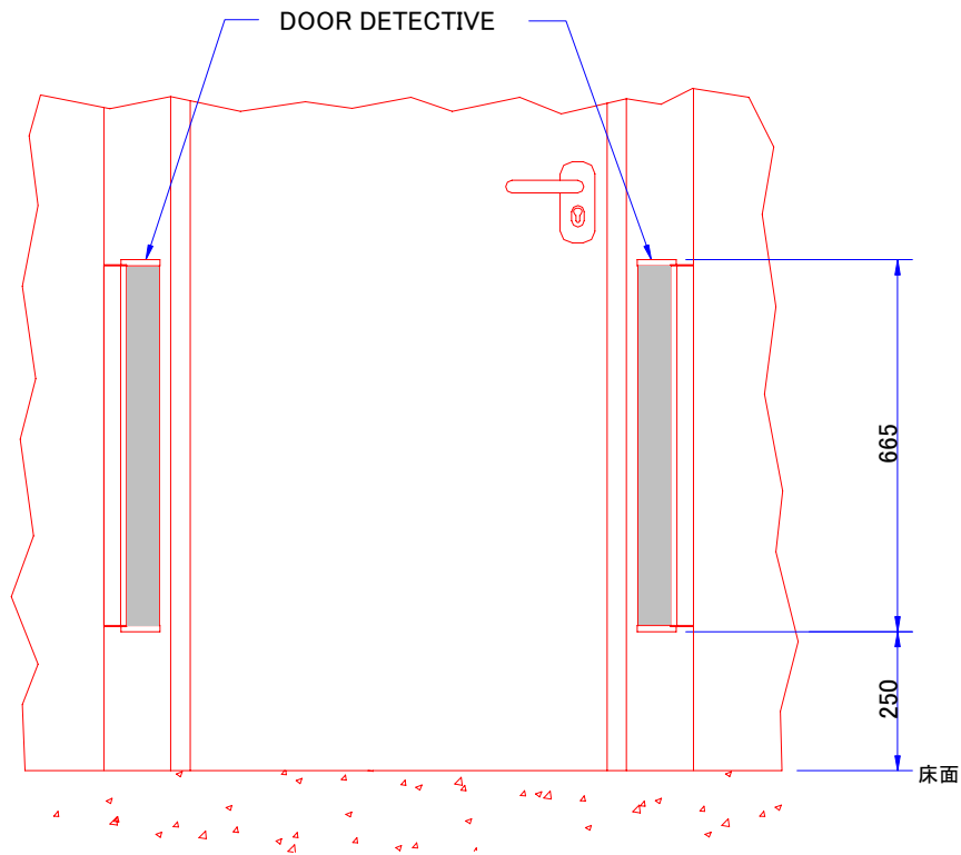
正面図
